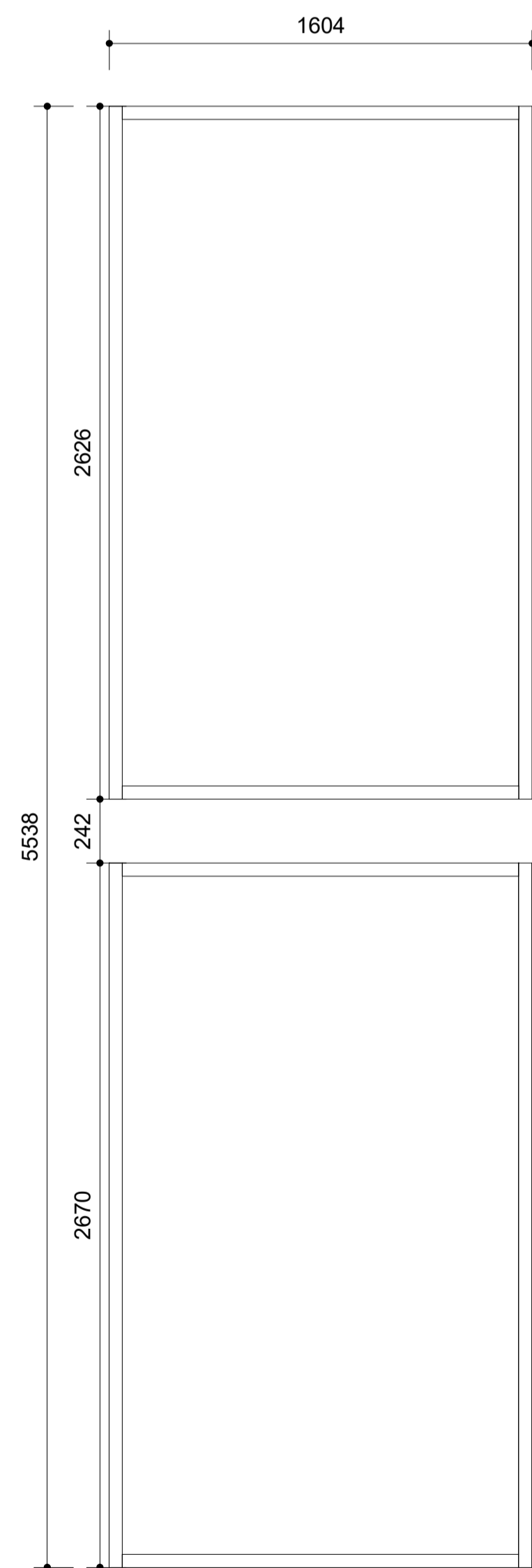
G12-D mkv: 1 : 20
